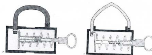
تصویر ۱۳: مکانیزم درونی قفل‌های چالستر با فنر مارپیچ (تناولی ۱۳۸۶، ۳۳).
